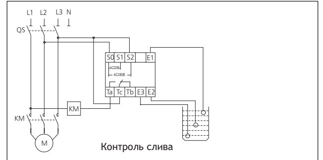
Для NJYW1-NL1, NJYW1-NL2 напряжение питания 220V/380В
