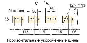
Горизонтальные укороченные шины
