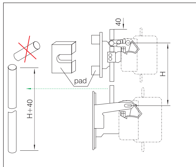
Схема установки контакторов
