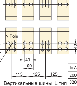
Вертикальные шины L тип
