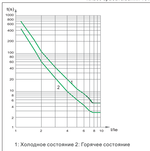
Класс срабатывания 10 A
