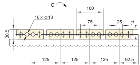
Горизонтальные укороченные шины
