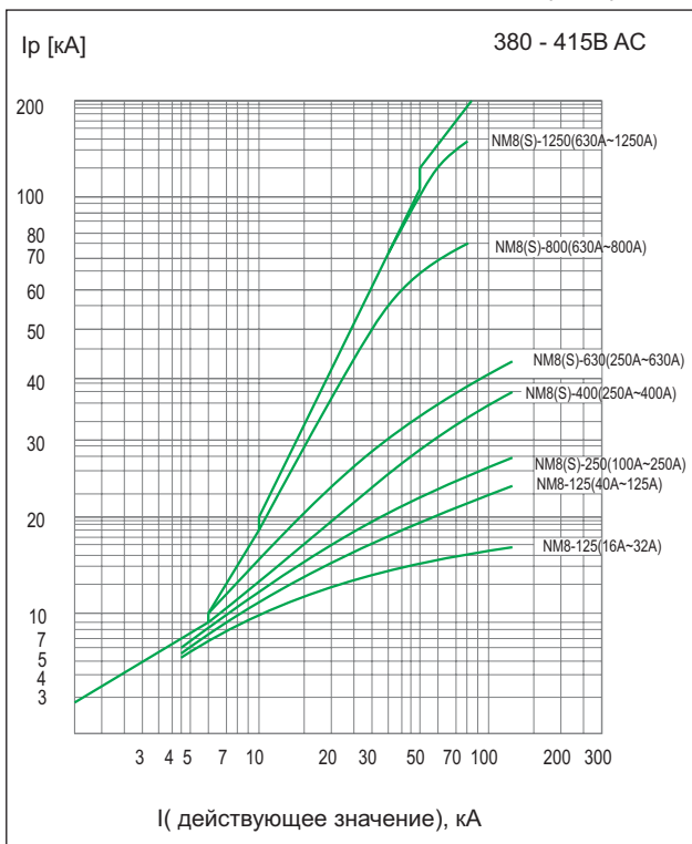
I^2 t характеристика
