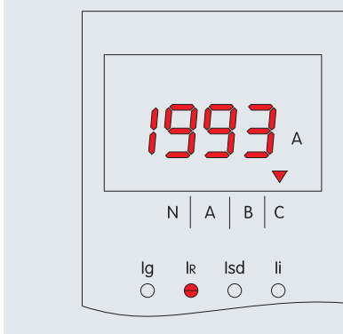
Состояние запроса о срабатывании - ток срабатывания
