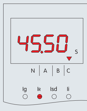
Состояние запроса о срабатывании - время срабатывания
