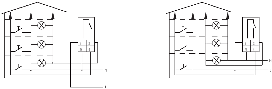
Электрическая схема NJS3 (3 провода)
