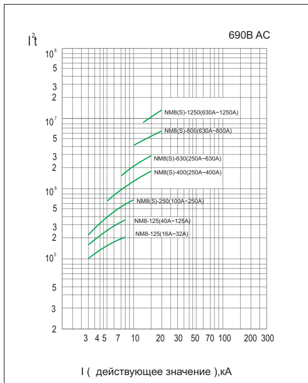
A^2 сек характеристика
