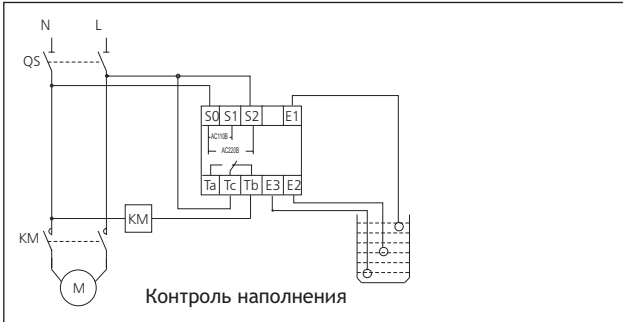
Для NJYW1-NL1, NJYW1-NL2 напряжение питания 110V/220В
